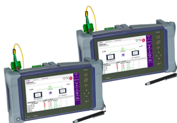
T-BERD/MTS-4000 V2
